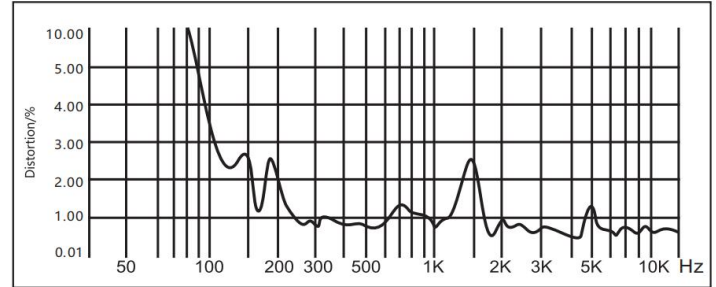
Distortion Characteristic (THD<5% 1W、1m、100Hz-10kHz)
